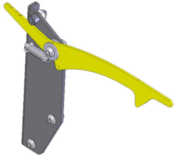
OAP824 - Mekaaninen kulkusillan lukitus DH-AI
