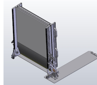
OAF820.L - Kääntyvä runko DHAI - V
